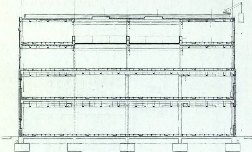
Sección, plantas baja, primera, segunda y tercera y alzados de la Sede para la Dirección de Renfe Section, ground, first, second and third floor, and elevations of the Renfe Administration Building
